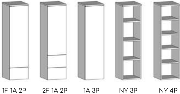
eTETRIS 150/40 150x40x42,5
